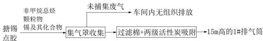
图 4.1-1 本项目废气处理装置收集方式
