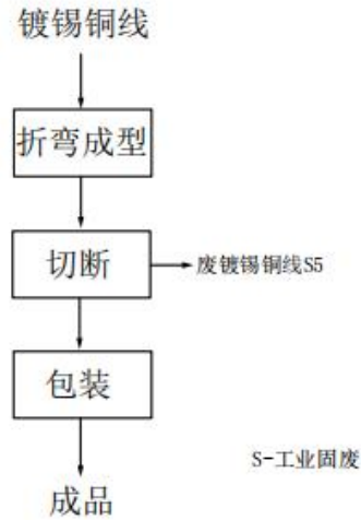
图 2-2 线桥工艺流程及产污节点图
