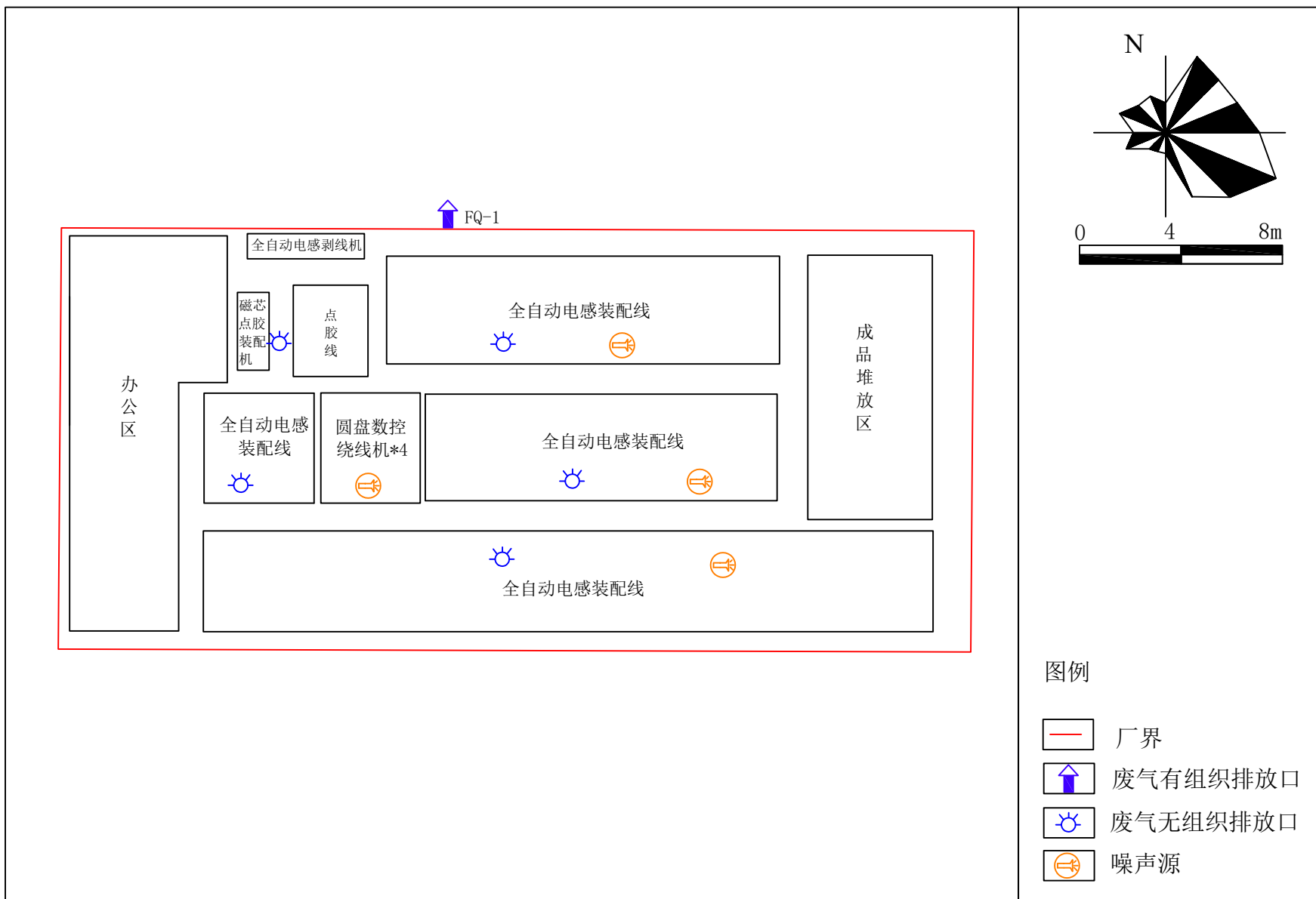
附图3-2 车间平面布置图（2F）
