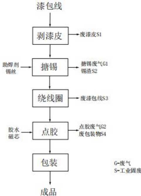
图 2-1 电感工艺流程及产污节点图
