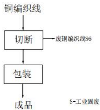
图 2-3 编织线桥工艺流程及产污节点
