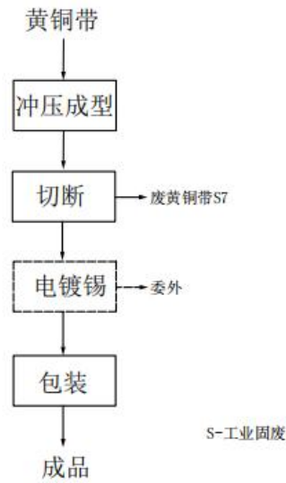
图 2-4 接线端子流程及产污节点
